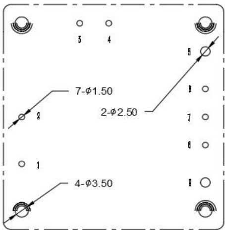
推荐PCB开槽尺寸
