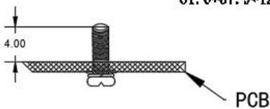
标准型 61.0*57.9*12.7mm
