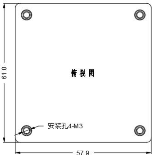
标准型 61.0*57.9*12.7mm
